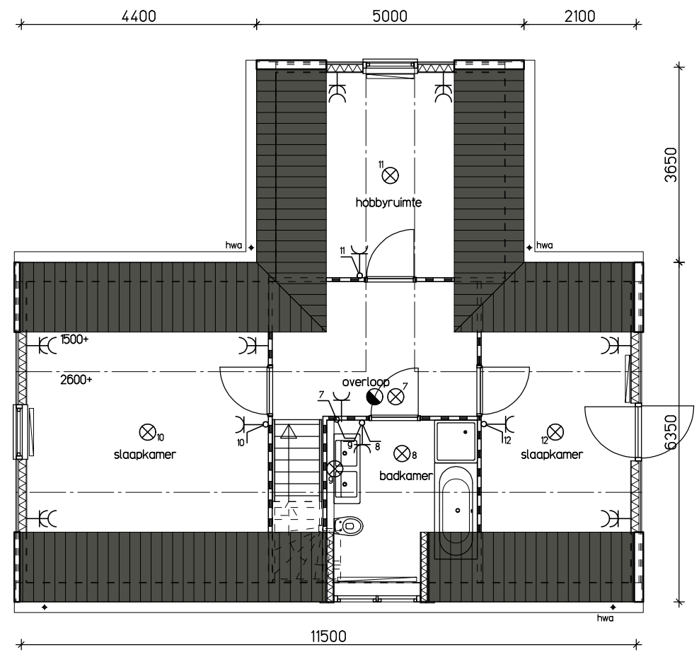
verdieping
