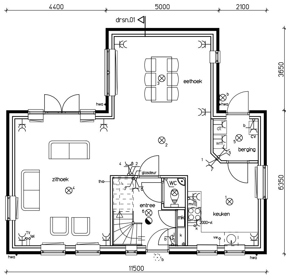
begane grond
