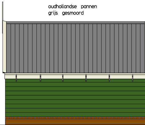
zijgevel links/rechts
